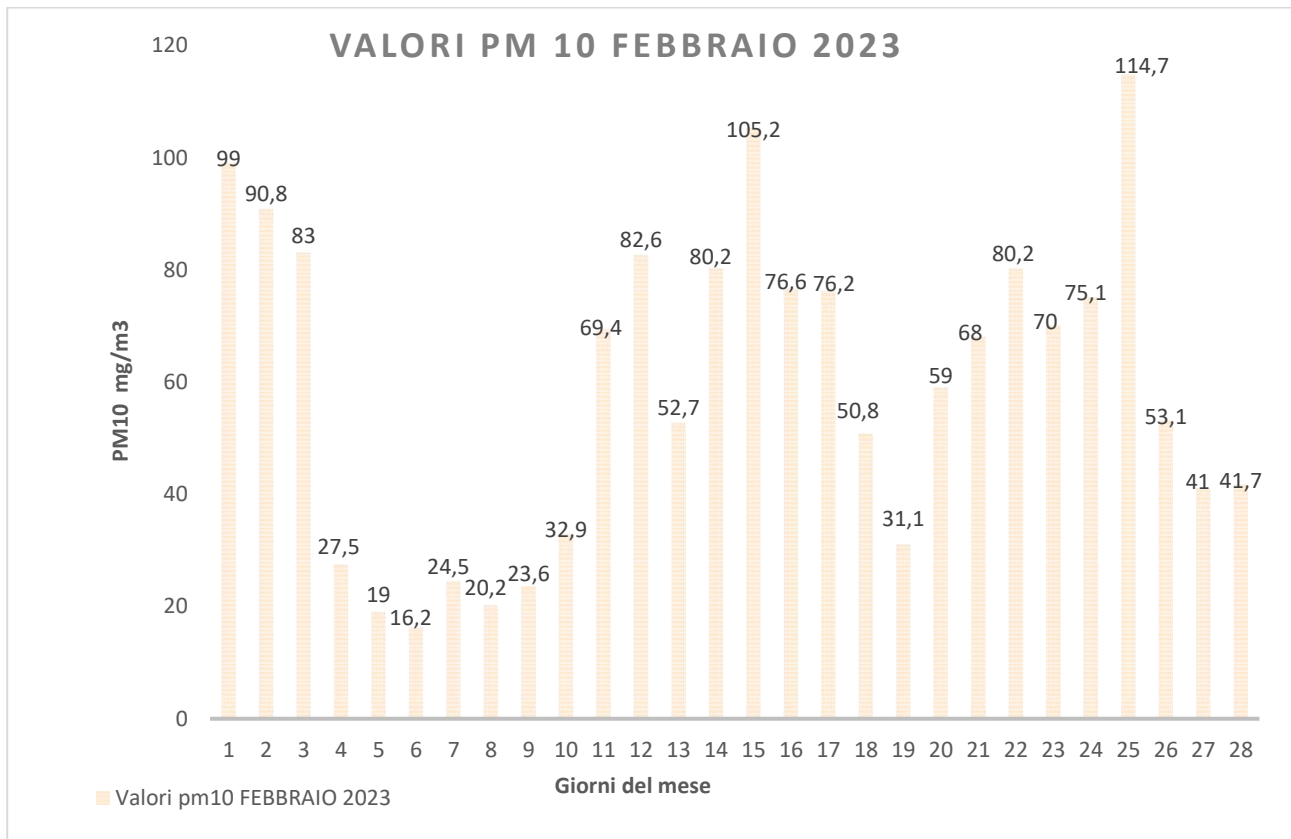
Grafico 1. Andamento polveri sottili PM10 mese di Febbraio 2023- Valori rilevati dalla centralina posizionata presso la Casa Comunale (Gestione Ufficio Ambiente)
